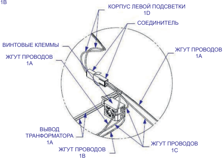
Деталь G
