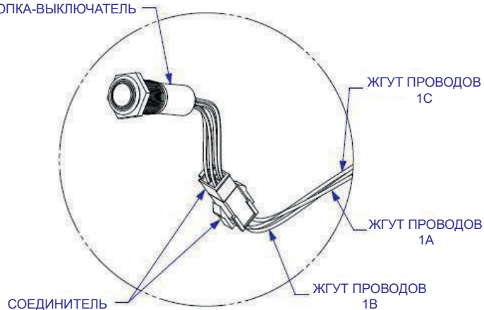
Деталь F
